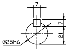
INPUT SHAFT
