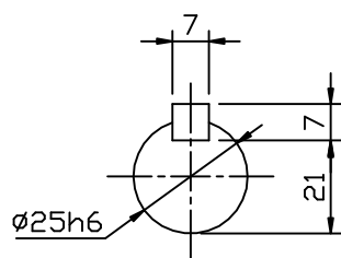
INPUT SHAFT
