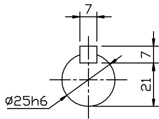
INPUT SHAFT
