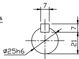
INPUT SHAFT
