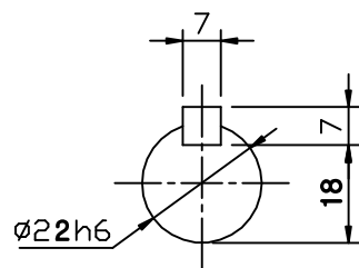
INPUT SHAFT
