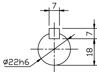
INPUT SHAFT
