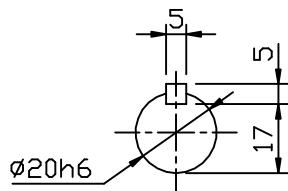
INPUT SHAFT
