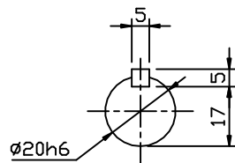
INPUT SHAFT
