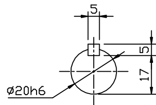
INPUT SHAFT
