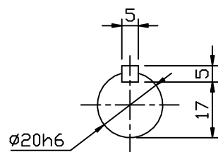
INPUT SHAFT
