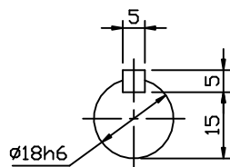
INPUT SHAFT
