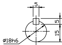
INPUT SHAFT
