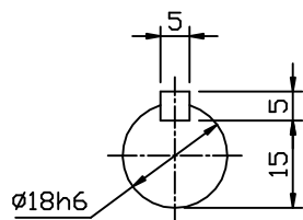
INPUT SHAFT
