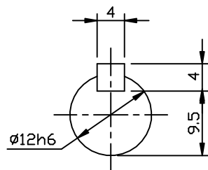
INPUT SHAFT
