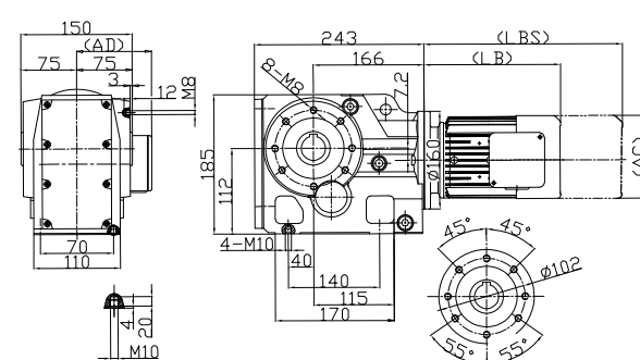
DKA47
