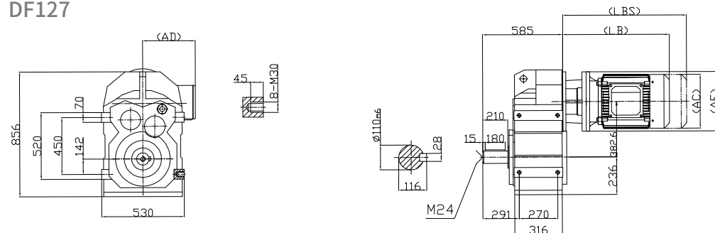
DF127
