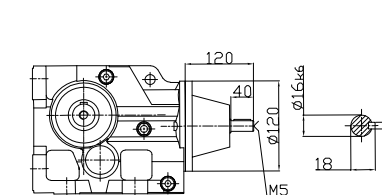
DK..S37
