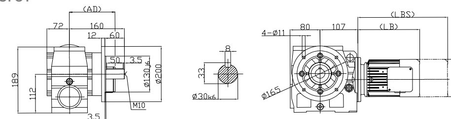
DSF57
