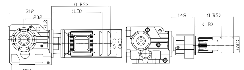
DK..77DR37
