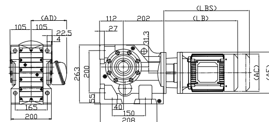
DKAB77
