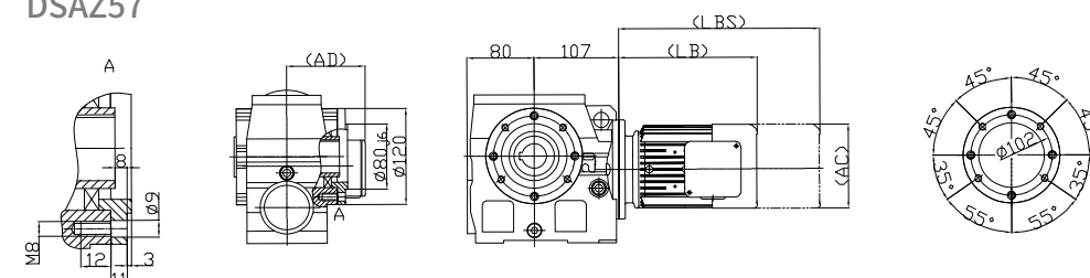
DSAZ57
