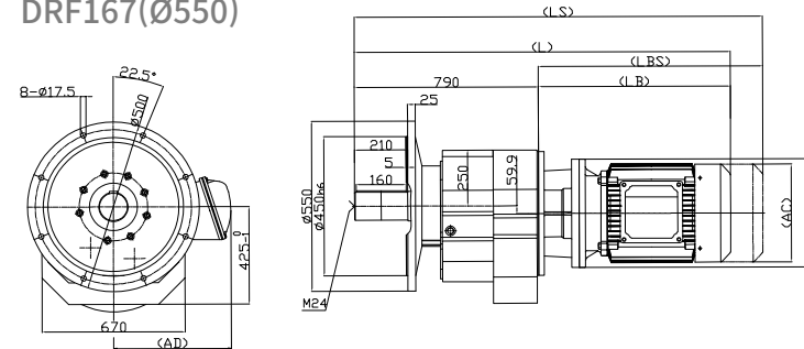
DRF167(Ø550)
