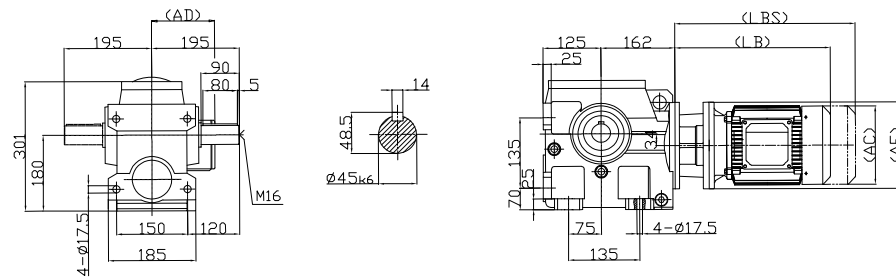
DSAT77
