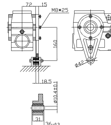
DSAT57
