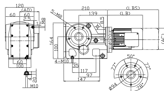
DKA37
