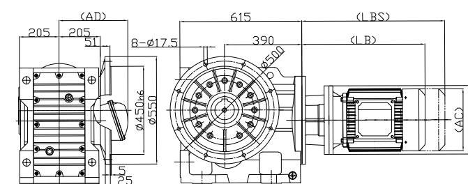
DKAF127
