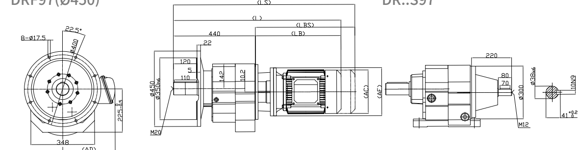
DRF97(Ø450)
