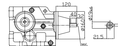
DK..S47
