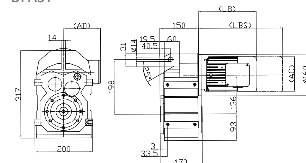
DFA57
