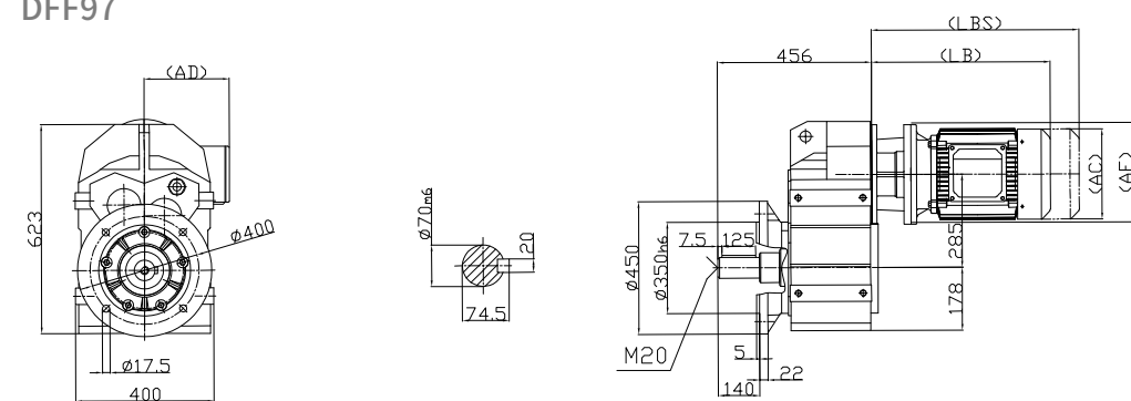
DFF97
