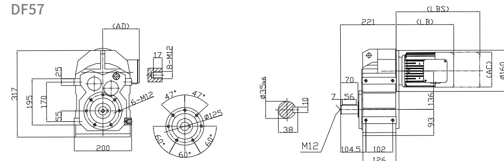
DF57
