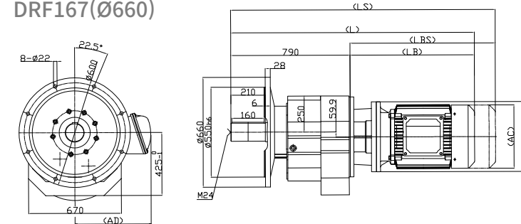
DRF167(Ø660)
