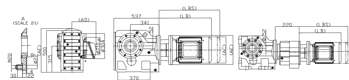
DKAZ107
