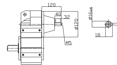
DF..S47
