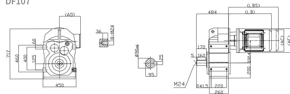
DF107
