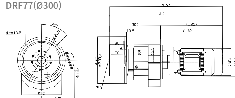
DRF77(Ø300)
