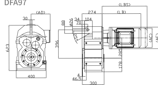
DFA97
