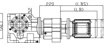
DK..107DR77
