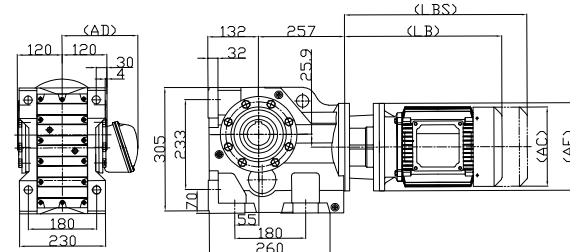
DKAB87
