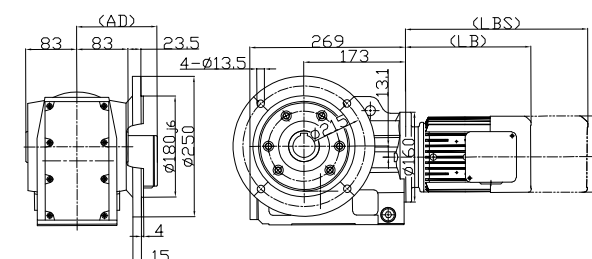
DKAF57
